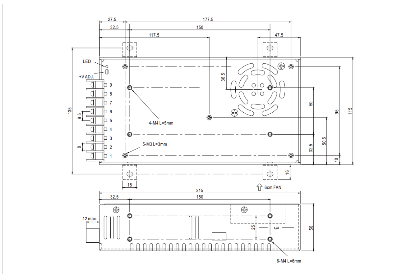
Рис. 1. Внешний вид импульсного блока питания
